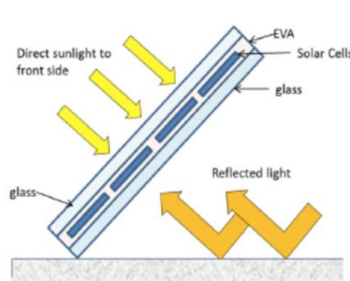
Bifacial module
