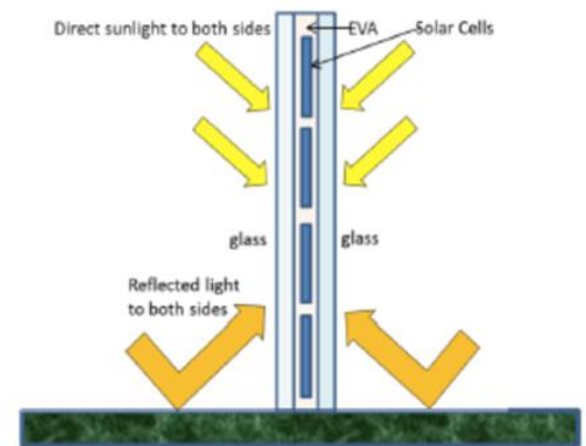
Bifacial module
