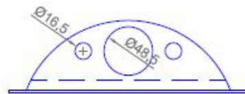
Solarluke ohne Tüllen mit Tülle max Ø 35mm/10mm
