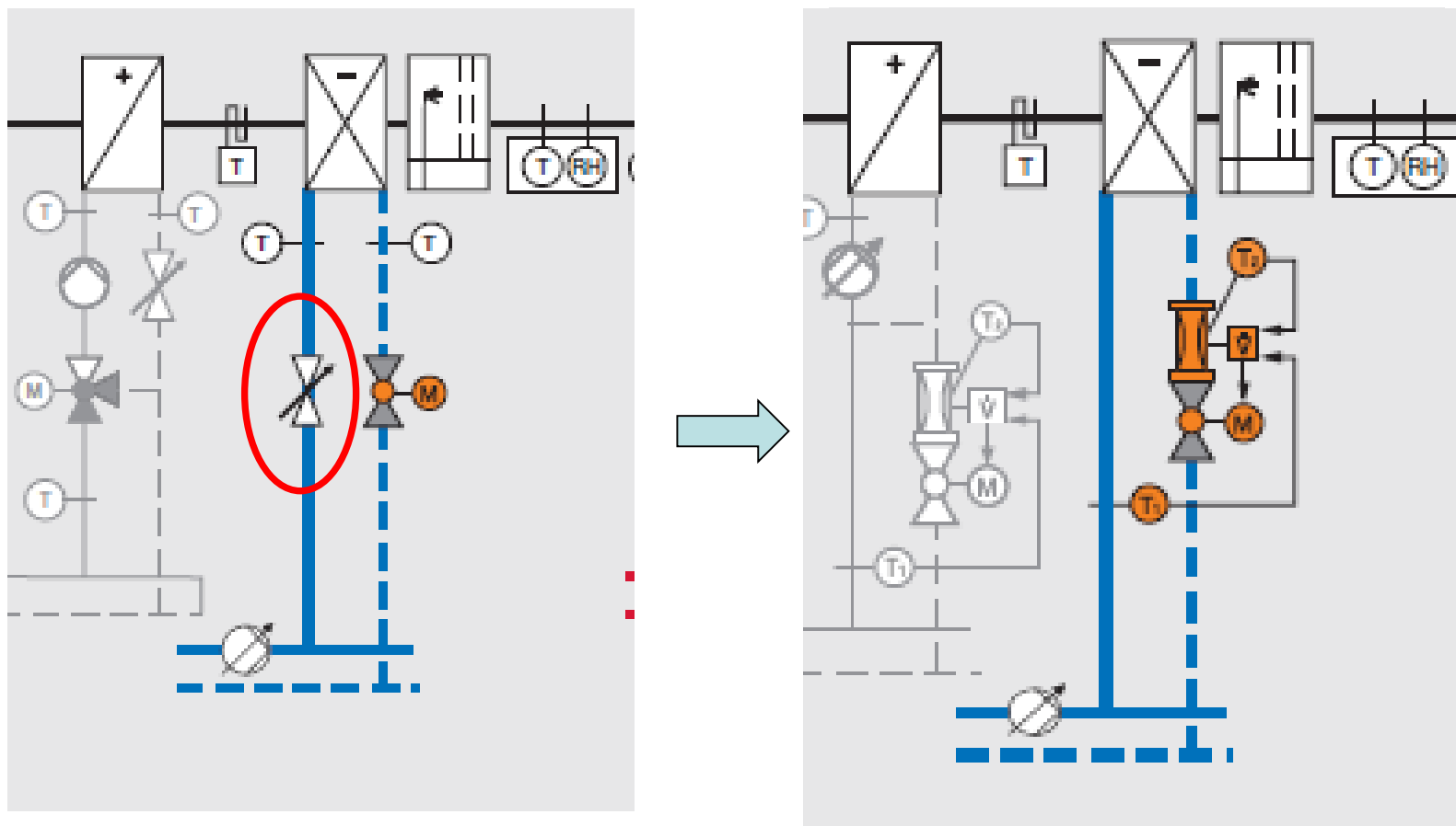
Nyomásfüggetlen rendszer – fojtó kapcsolás
