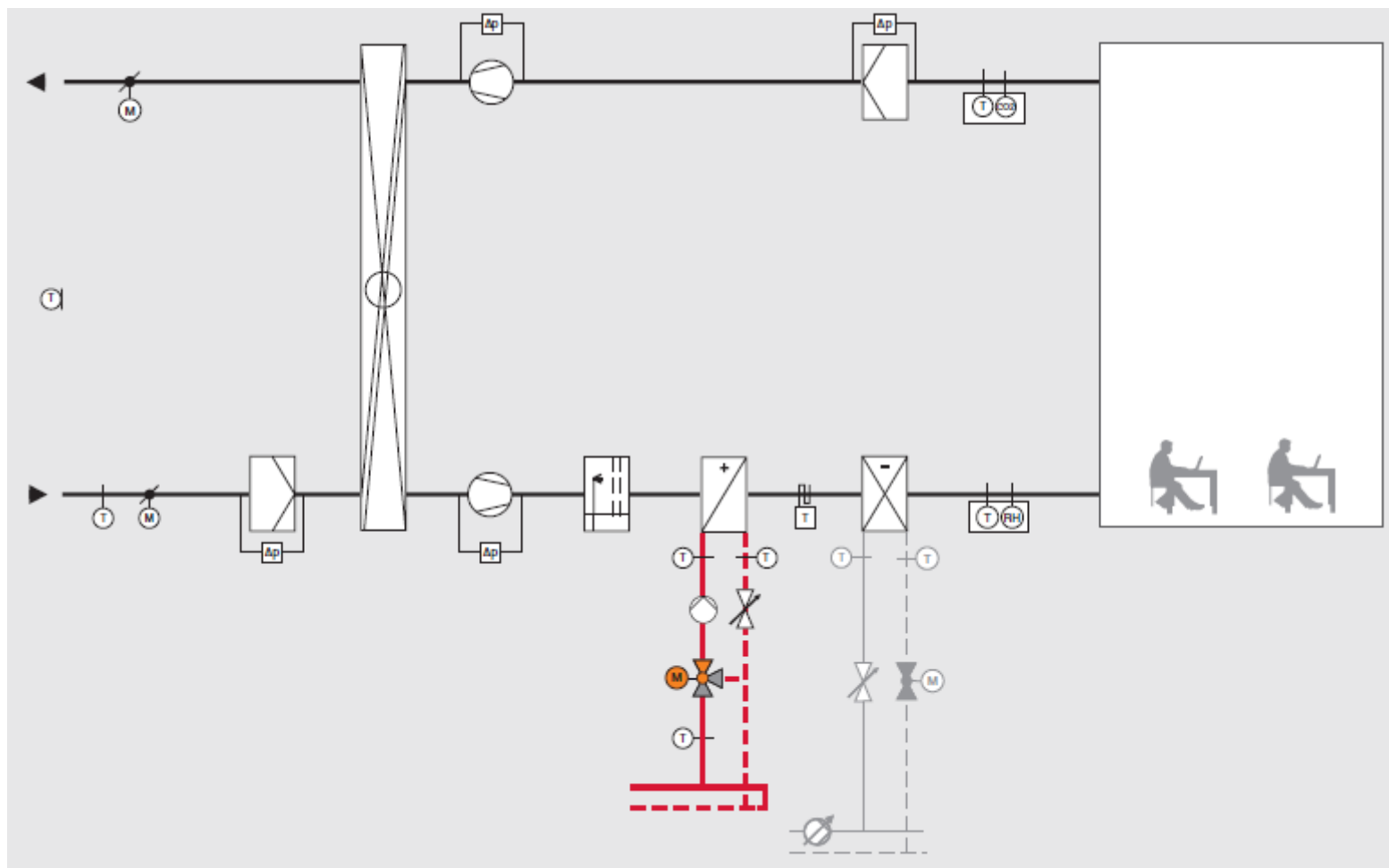
Nyomásfüggő rendszer – keverő kapcsolás
